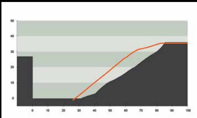
Profilé, corps N° 28 / N° 9 Profondeur : 26 cm, largeur de semelle 30 cm, largeur 73 cm
