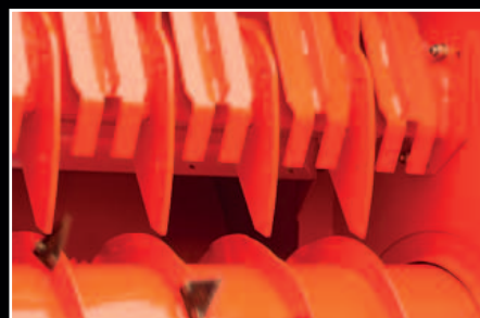
Un brevet KUBOTA – DFCS désengagé pour un flux maximum vers la turbine.
